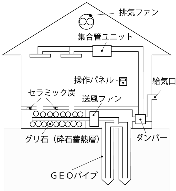
【地中熱利用のジオパワーシステムの概略図】
